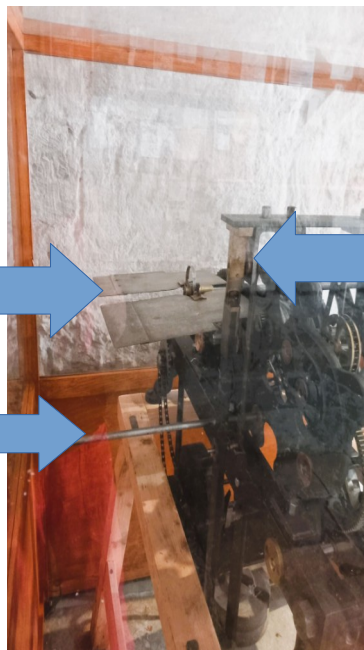
Le câble qui relie le poids de 50kg au mécanisme
